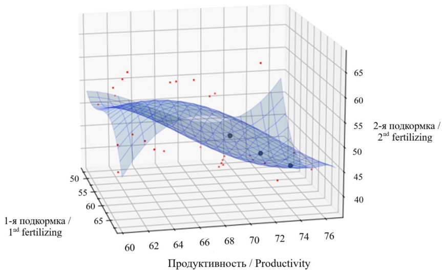
Р и с. 7. Трехмерная квадратичная плоскость
