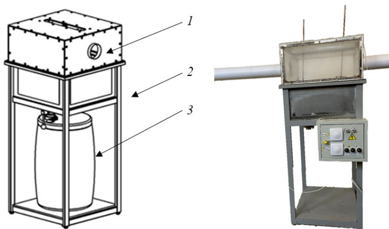
Р и с. 1. Общий вид разработанной экспериментальной установки: 1 – герметичная камера; 2 – каркас; 3 – емкость для слива жидкой фракции навоза
