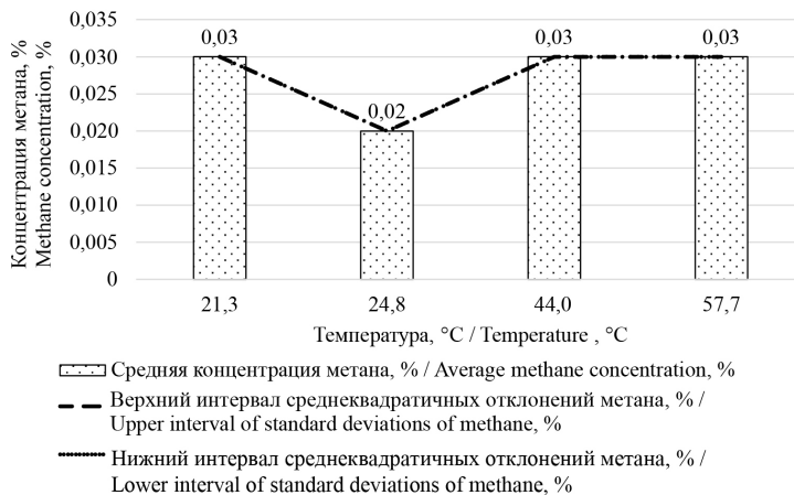
Р и с. 5. Значения средней концентрации метана, верхний и нижний интервалы средноквадратических отклонений метана
